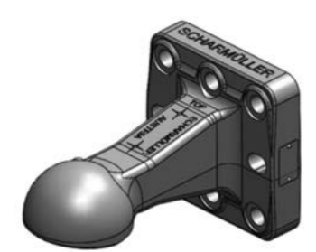
hemisphere Ø80
